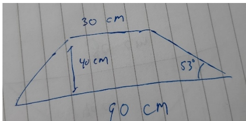
Figur 2 Tværsnit af dige
